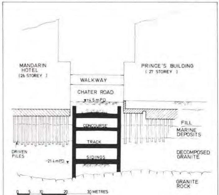
Fig. 4 Section 2-2
