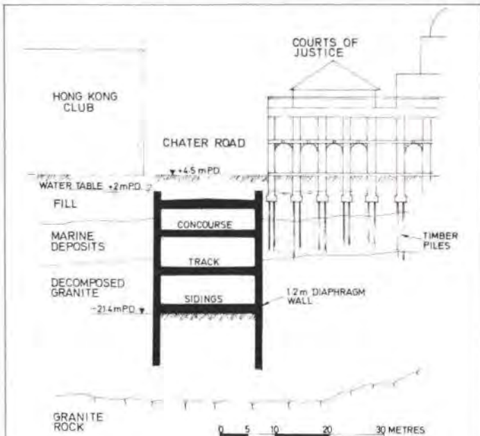
Fig. 3 Section 1-1
